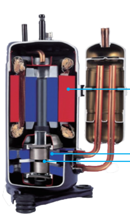
Компрессор (двухроторный)
