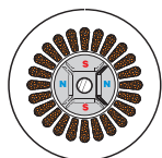
Централизованная обмотка
